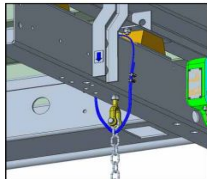
프레임(FRAME) 일체형 (동일부재에 체결)
