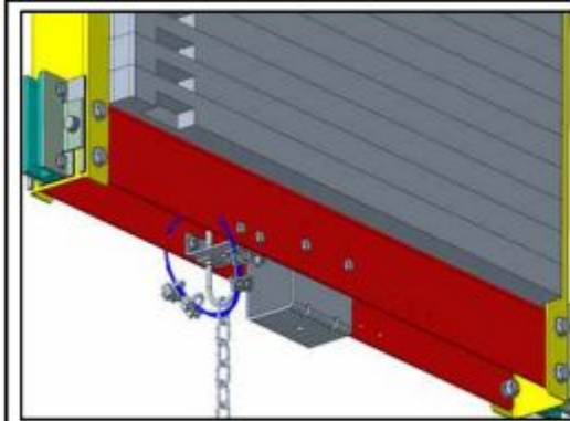
플레이트(PLATE) 용접형 등의 별도 부재 (U-BOLT와 다른 부재에 체결)
