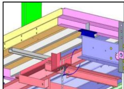
프레임(FRAME) 일체형이 아닌 경우 (프레임에 추가 연결)
